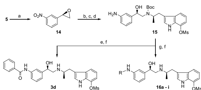
Scheme 4. Reagents: (a) 2 N NaOH, THF; (b) 7 , DMF; (c) (Boc) 2 O, CHCl_3 ; (d) Fe, NH_4Cl , EtOH, H_2O ; (e) PhCOCl , Et_3N , CHCl_3 ; (f) 4 N HCl–AcOEt; (g) R–Br, K_2CO_3 or Et_3N , DMF.
